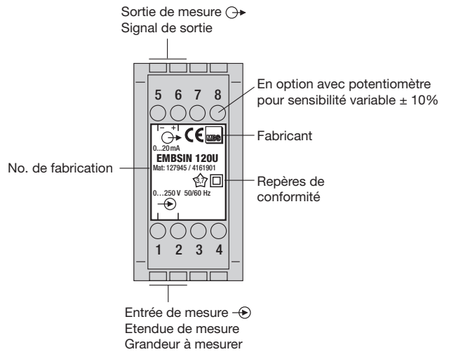
Fig. 3. Déclaration pour la plaquette signalétique.
