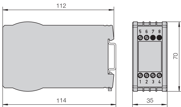
Bild 5. Gehäuse MBS/SP1 auf Hutschiene (35 × 15 mm oder 35 × 7,5 mm) nach EN 50 022.
