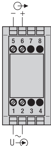
Fig. 2. EMBSIN 120 U, pour mesure de la tension alternative.
