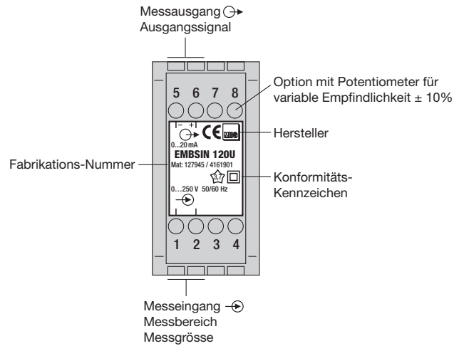
Bild 3. Erklärungen zum Typenschildbeispiel.
