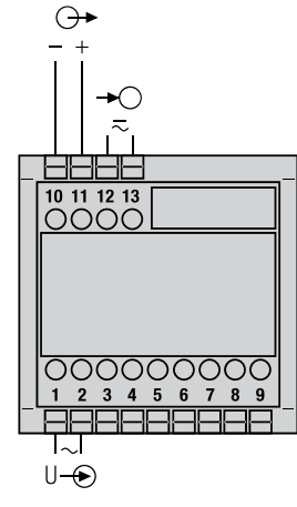
Bild 3. Hilfsenergie-Anschluss auf Niederspannungsseite an Klemmen 12 und 13.
