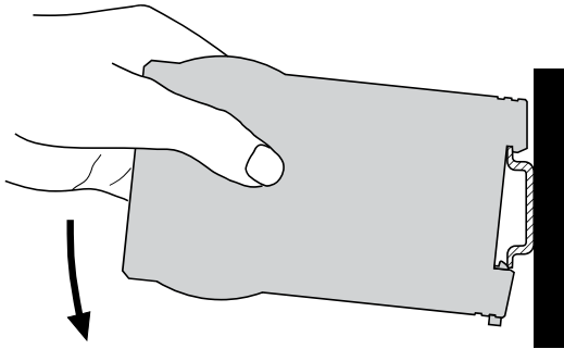
Bild 1. Montage auf Hutschiene 35 × 15 oder 35 × 7,5 mm.
