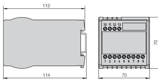
Fig. 8. Boîtier type MBS/SP2 encliqueté sur rail «à chapeau» (35 × 15 mm ou 35 × 7,5 mm, selon EN 50 022).
