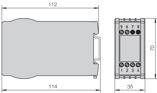
Bild 6. Gehäuse MBS/SP1 auf Hutschiene (35 × 15 mm oder 35 × 7,5 mm) nach EN 50 022.
