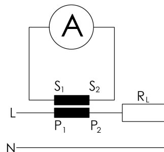
Messschaltung
