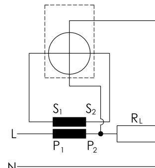
Zählerschaltung, einphasig
