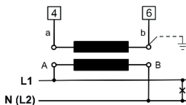
Wandlerschaltung
