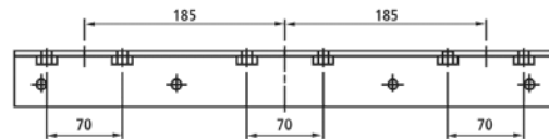
Halter L185/2 (2 x M10 je Phase)
