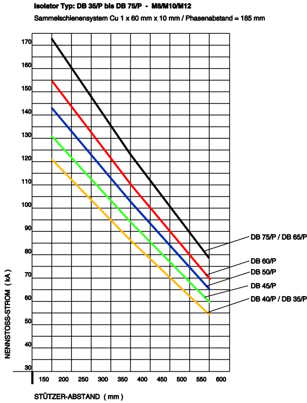
KURZSCHLUSSFESTIGKEIT / STÜTZERABSTAND - Tab. 3
