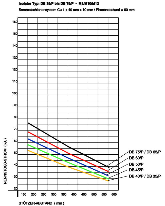
KURZSCHLUSSFESTIGKEIT / STÜTZERABSTAND - Tab. 4
