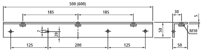
Halter L185/2 (2 x M10 je Phase)
